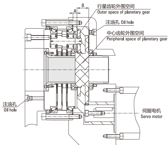
● 图 D.6: 润滑油注入位置(水平)
